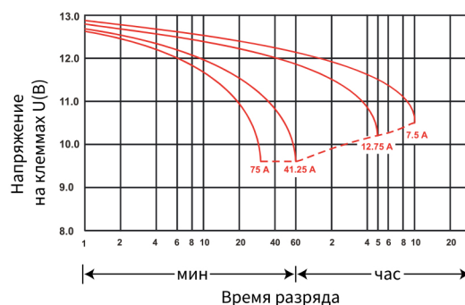
Разрядные характеристики
